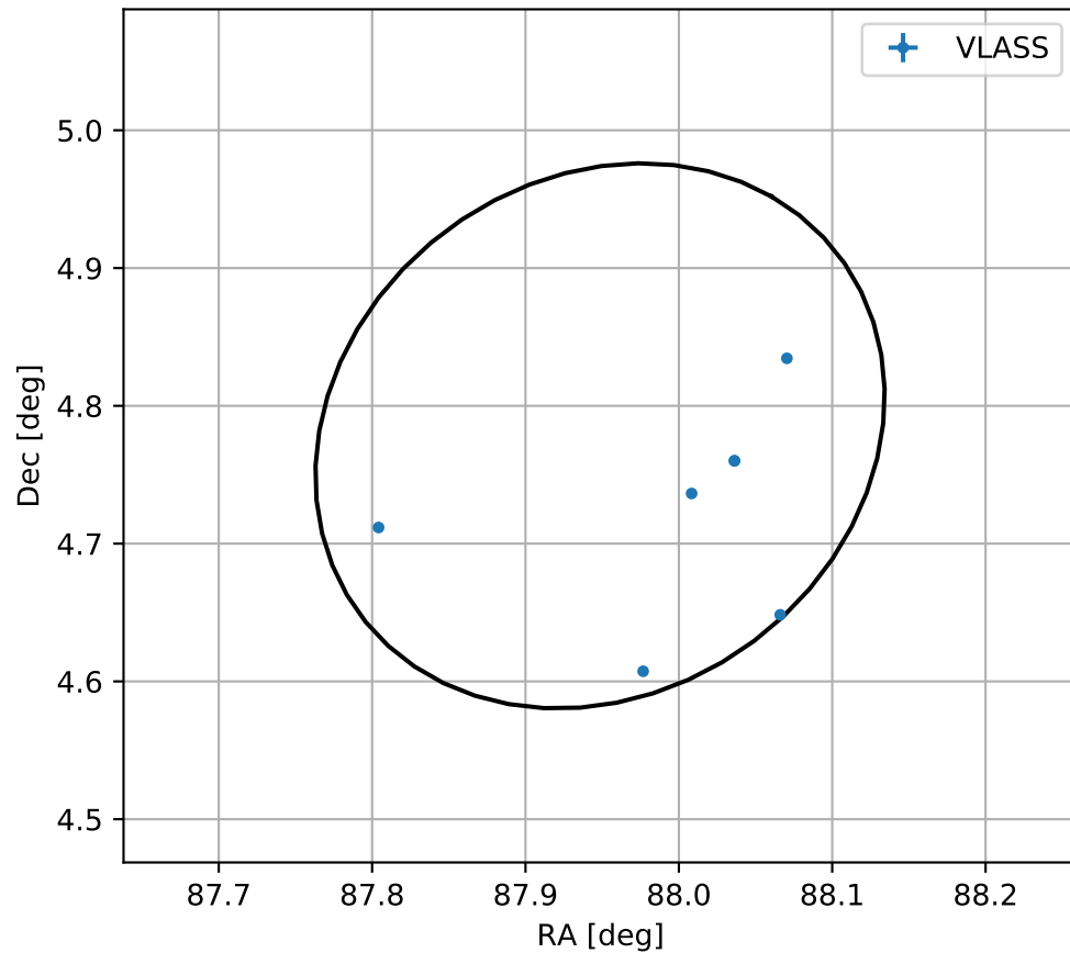
4FGL J0551.7+0446
