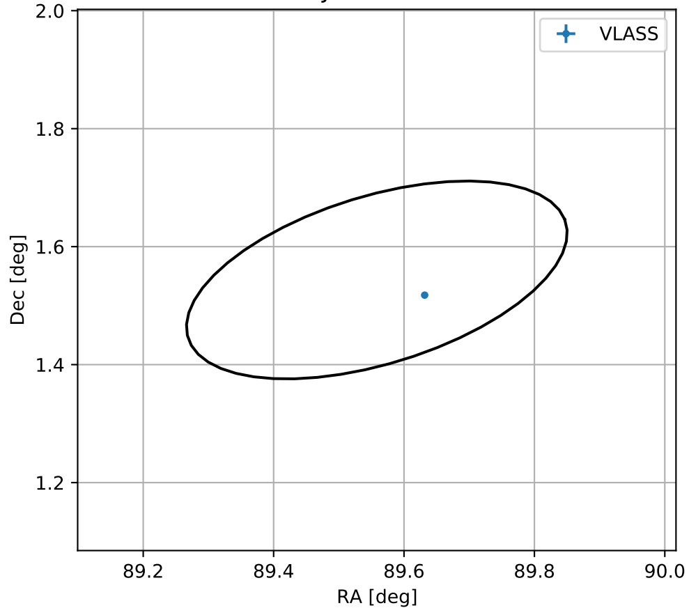
4FGL J0558.2+0132c
