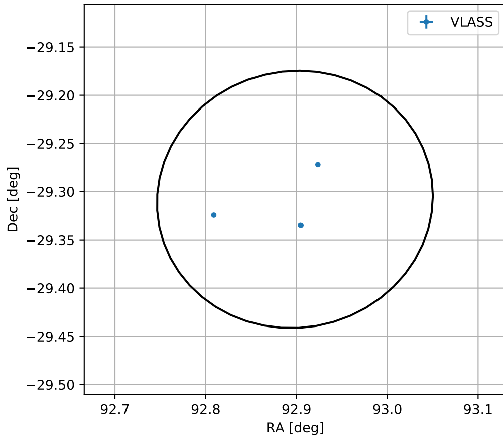
4FGL J0611.5-2918
