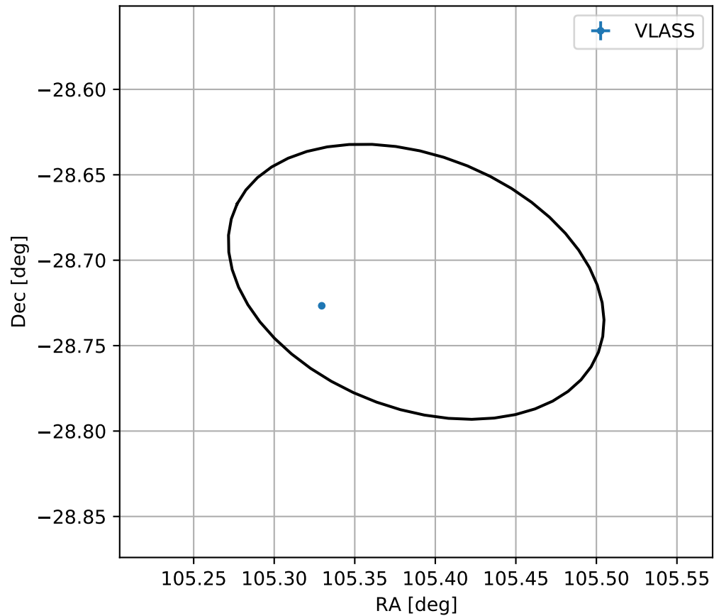
4FGL J0701.5-2842
