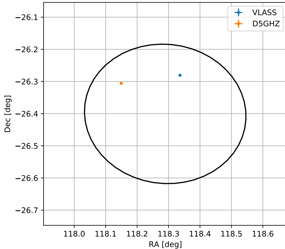
4FGL J0753.1-2624c
