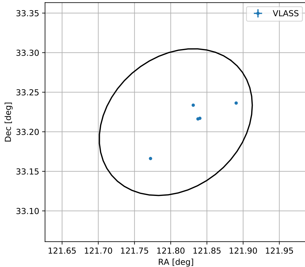
4FGL J0807.2+3312
