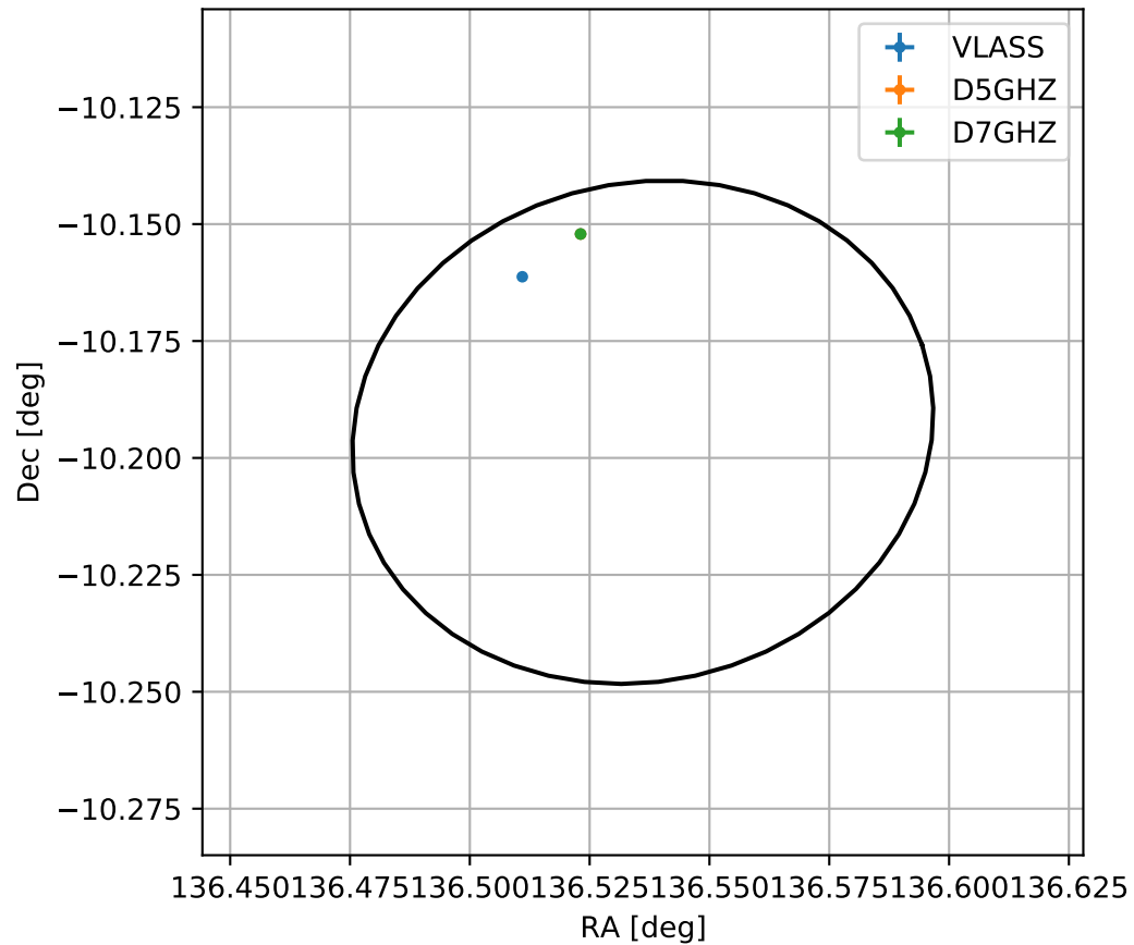
4FGL J0906.1-1011
