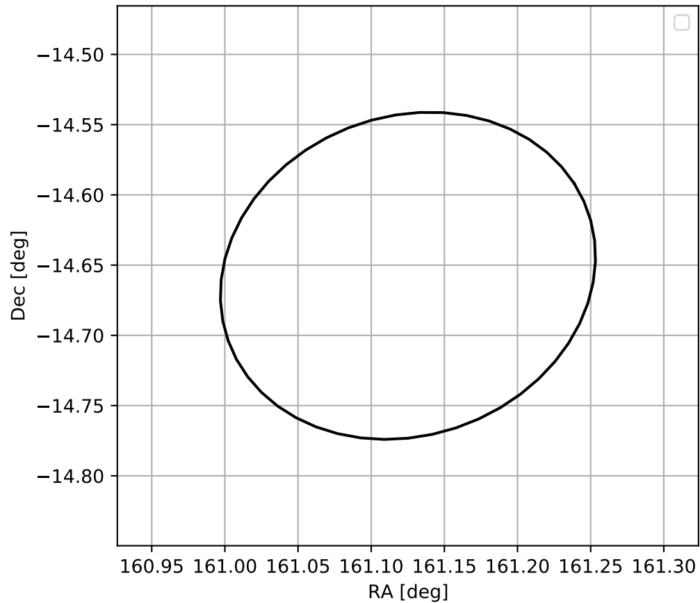
4FGL J1044.5-1439
