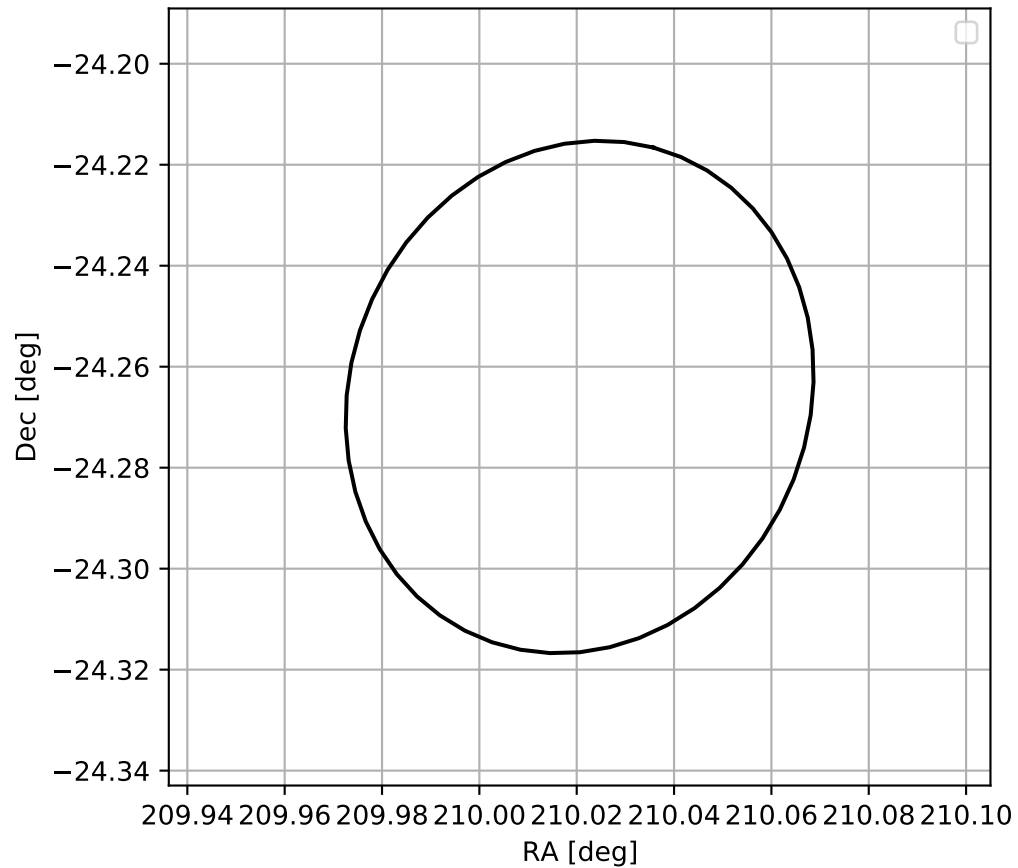
4FGL J1400.0-2415
