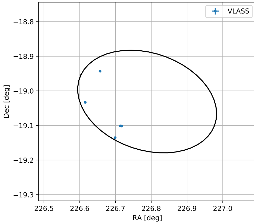
4FGL J1507.1-1901
