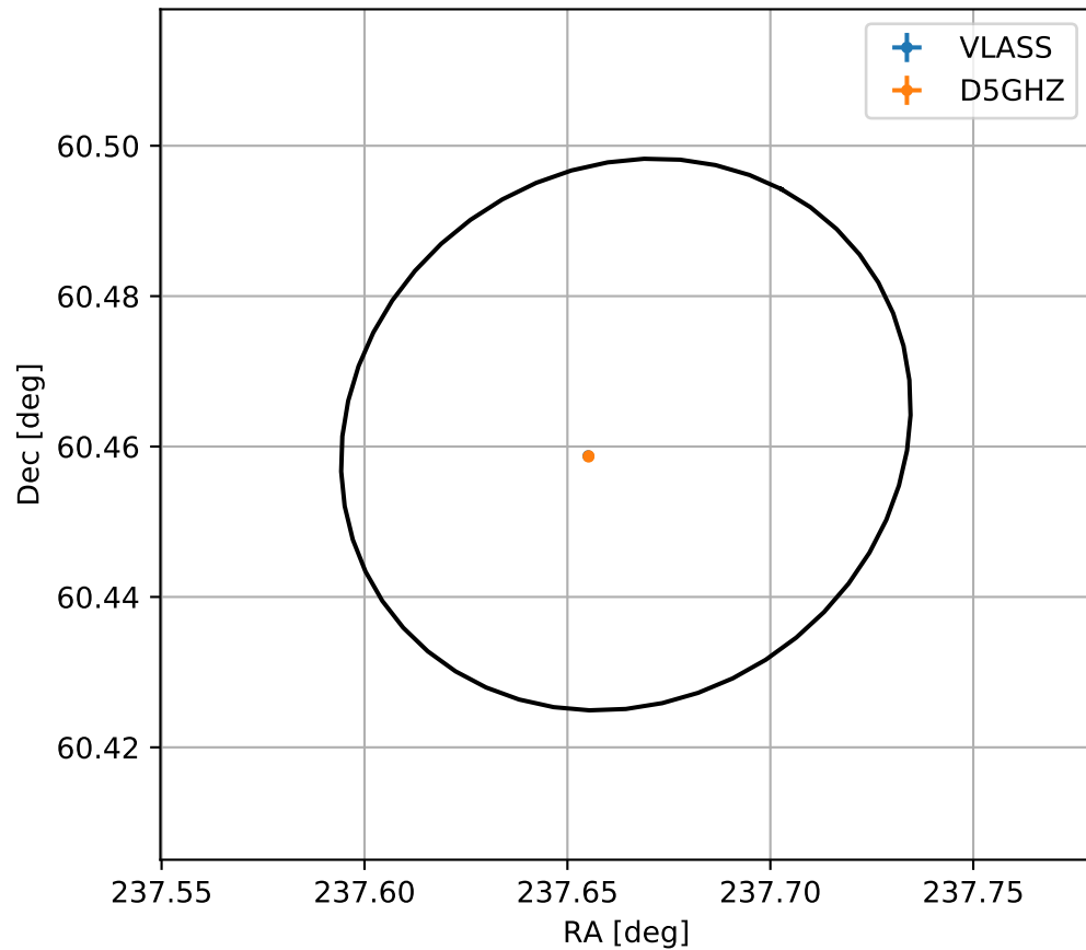
4FGL J1550.6+6027
