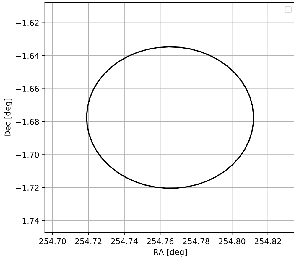
4FGL J1659.0-0140
