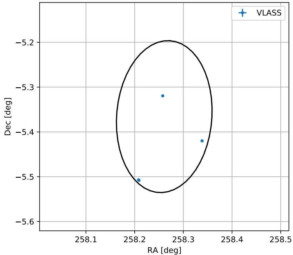
4FGL J1713.0-0521
