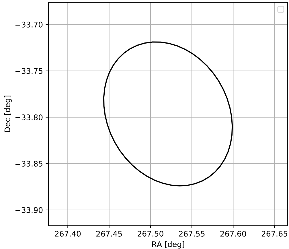
4FGL J1750.0-3347
