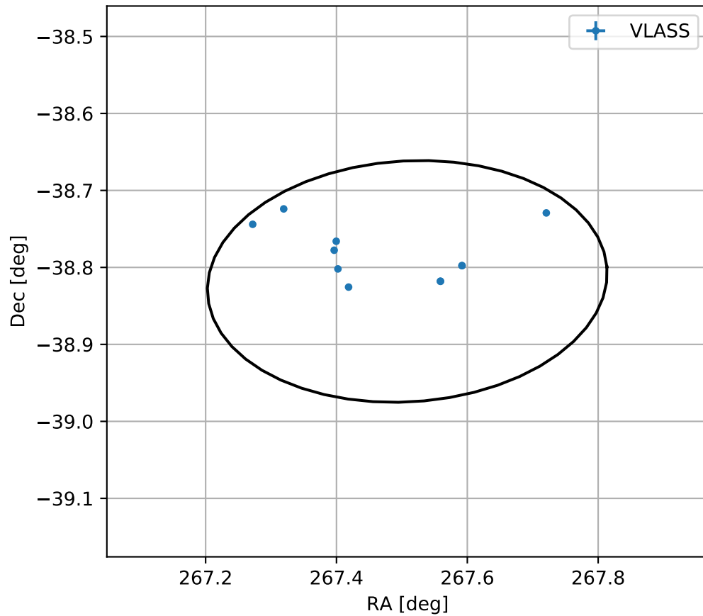
4FGL J1750.0-3849
