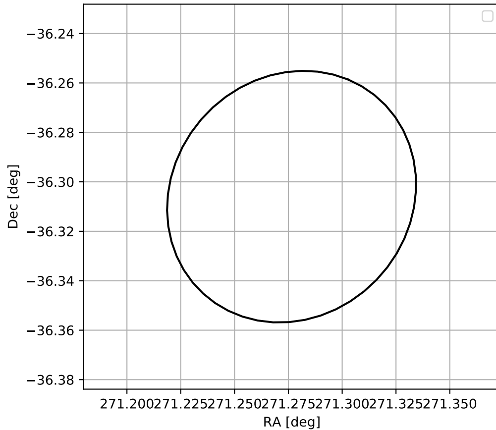
4FGL J1805.1-3618
