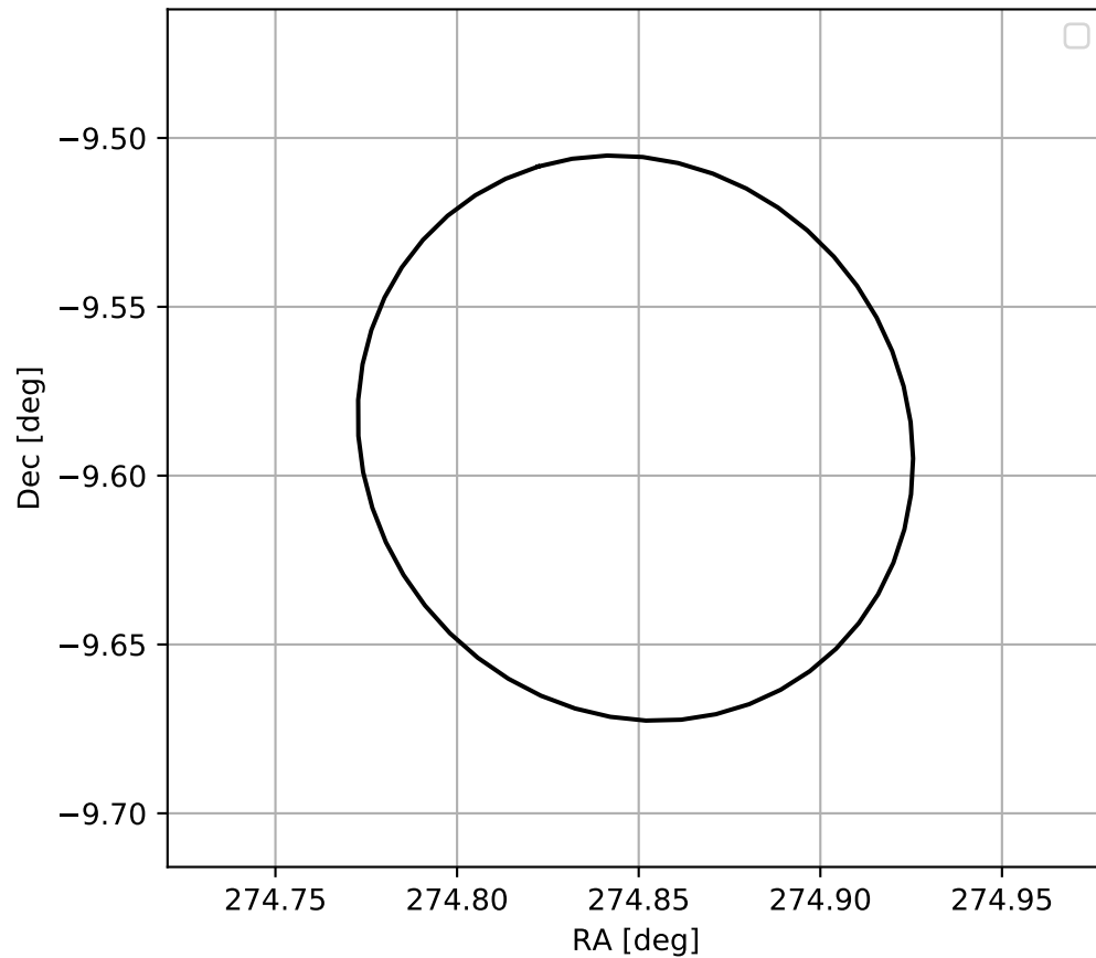
4FGL J1819.3-0935
