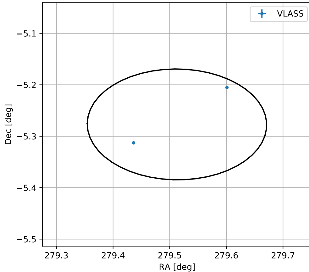
4FGL J1838.0-0516
