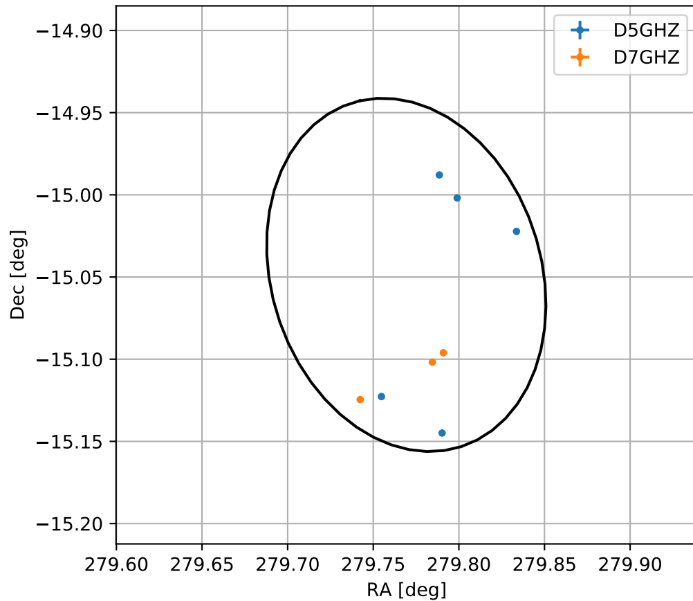
4FGL J1839.0-1502
