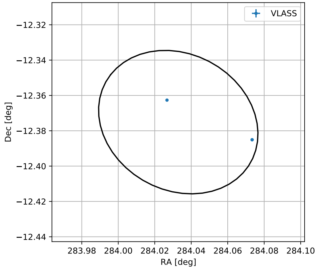
4FGL J1856.1-1222
