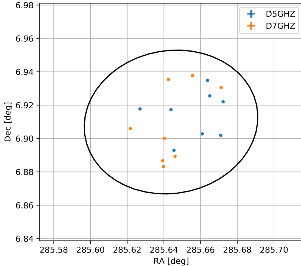
4FGL J1902.5+0654
