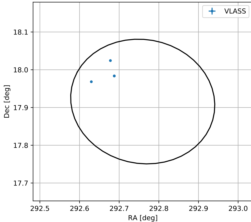
4FGL J1931.0+1754c
