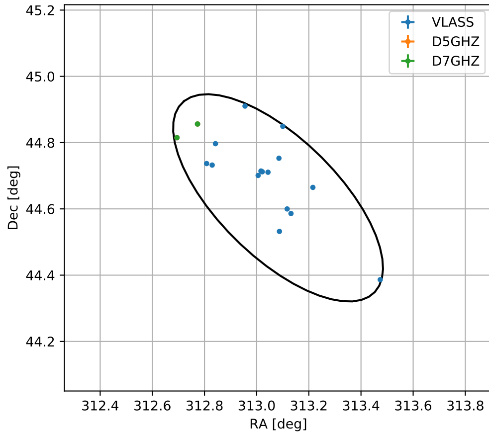
4FGL J2052.3+4437
