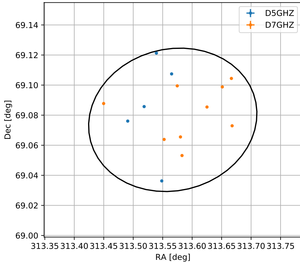
4FGL J2054.2+6904
