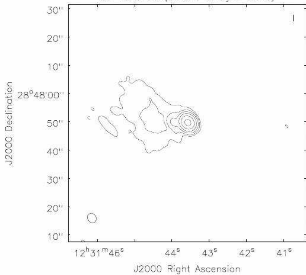
B2 1229+29 (JVLA B-array L-band)
