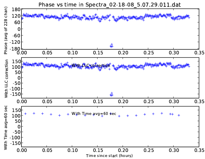
Fig. 4.— 0359 Xref=VaPax+15, Yref=VaPay-15, Zref=VaPaz+15
