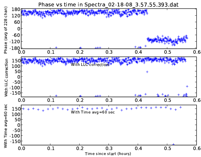
Fig. 2.— 0359 Xref=VaPax +15, Yref=VaPay, Zref=VaPaz
