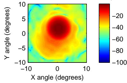
2007_Scan_13_Beam_2_FF.csv: amp
