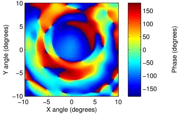
2007_Scan_17_FF.csv: phase
