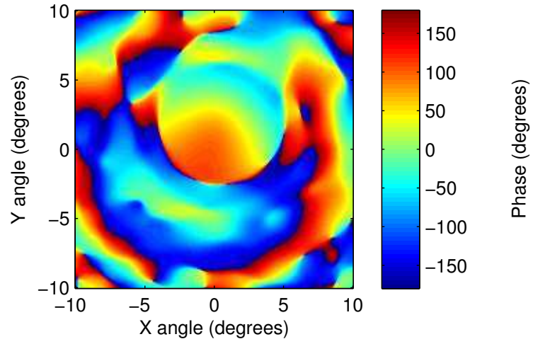
2008_Scan_8_FF.csv: phase
