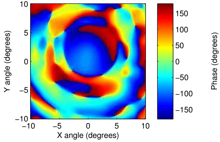
2007_Scan_11_FF.csv: phase
